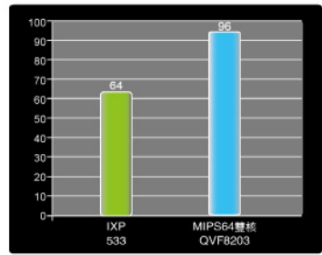
64Byte小包轉發效能 單位: Mbps
