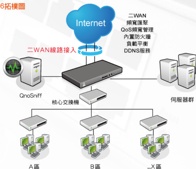
FQR8036拓樸圖
